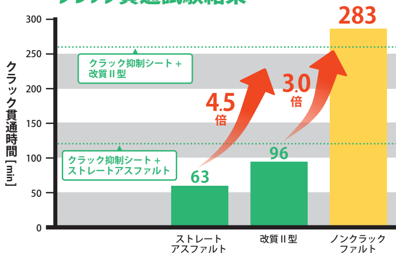
クラック貫通試験結果
