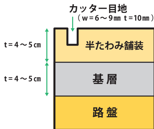
施工表面
