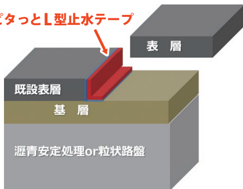
ピタッとL型止水テープ設置図
